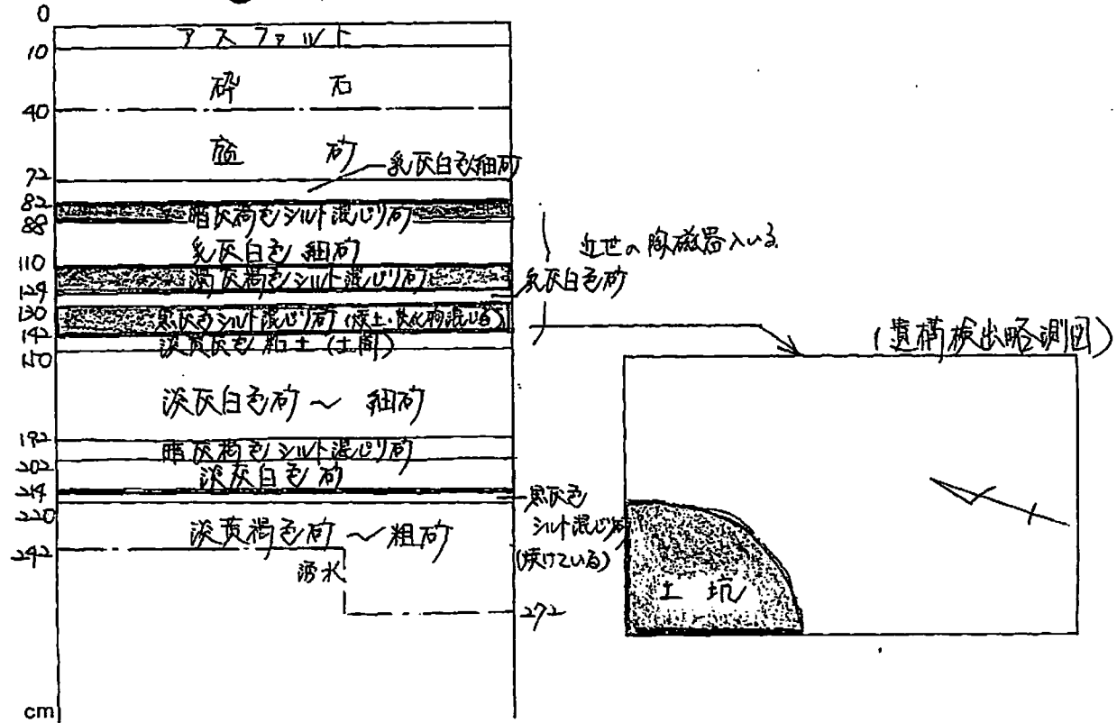
3 東壁断面
