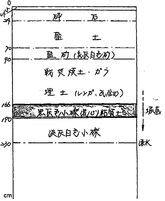
2 西壁断面
